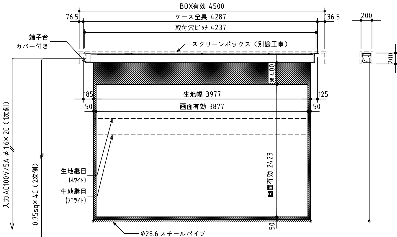
外観図 S=1/40
