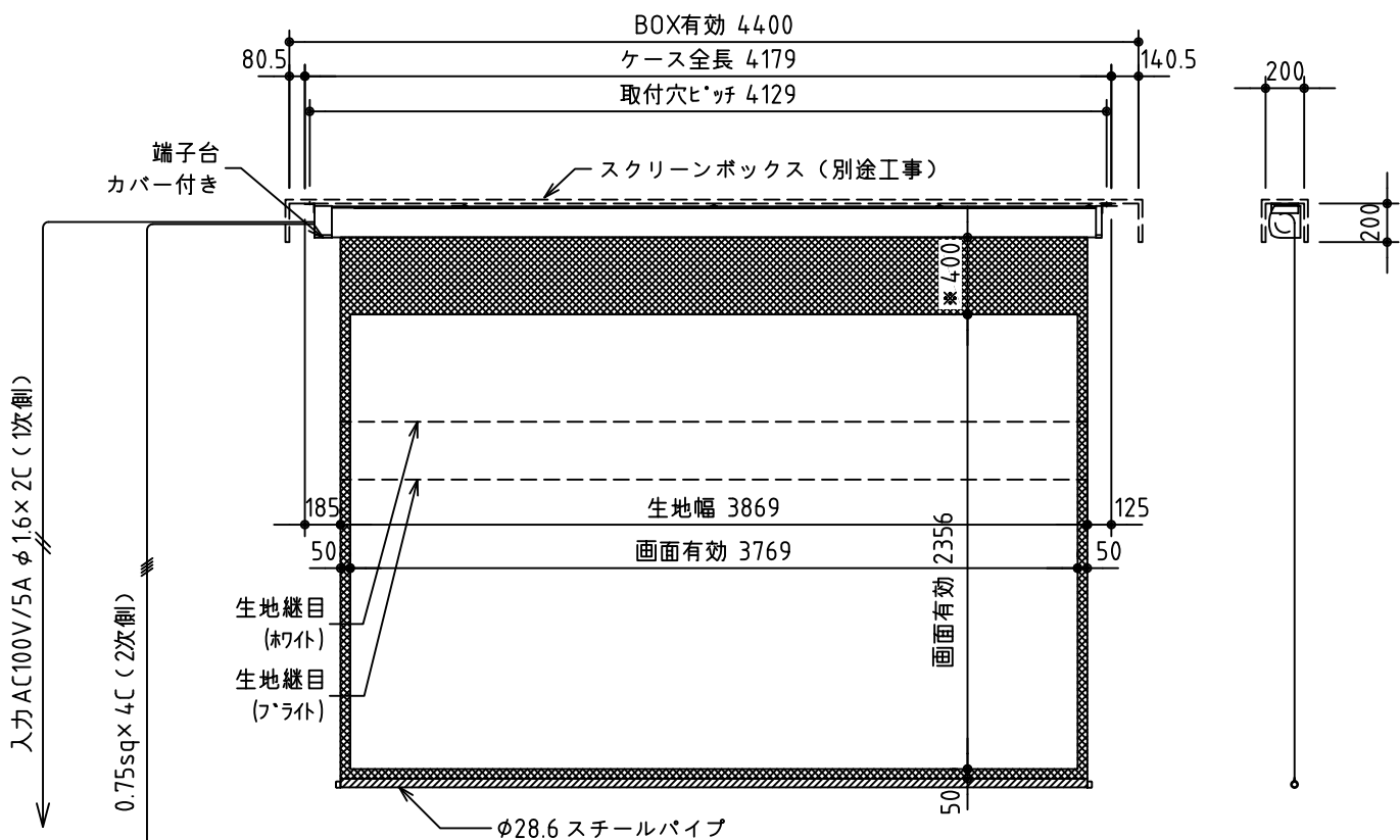
外観図 S=1/40
