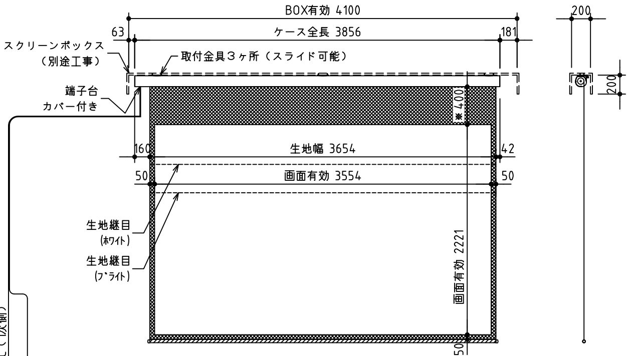
外観図 S=1/40
