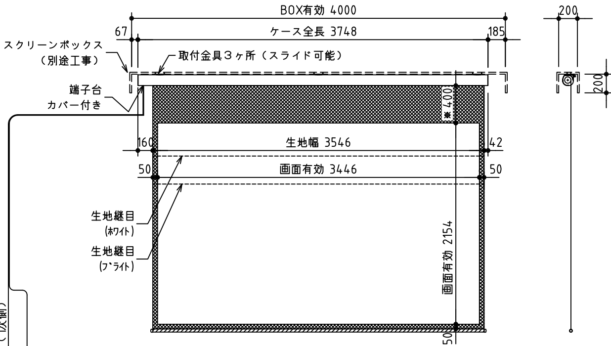
外觀図 S=1/40
