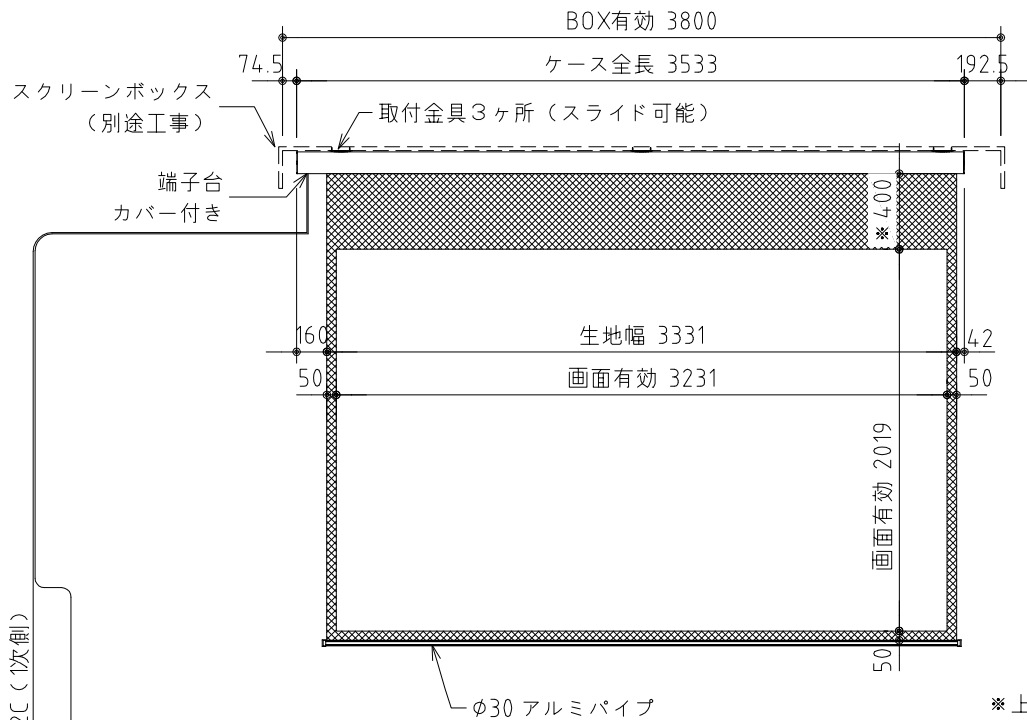
外観図 S=1/40
