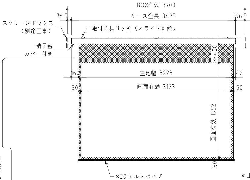
外観図 S=1/40
