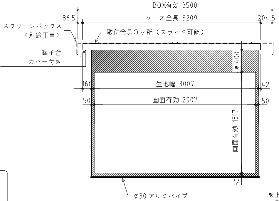
外觀図 S=1/40
