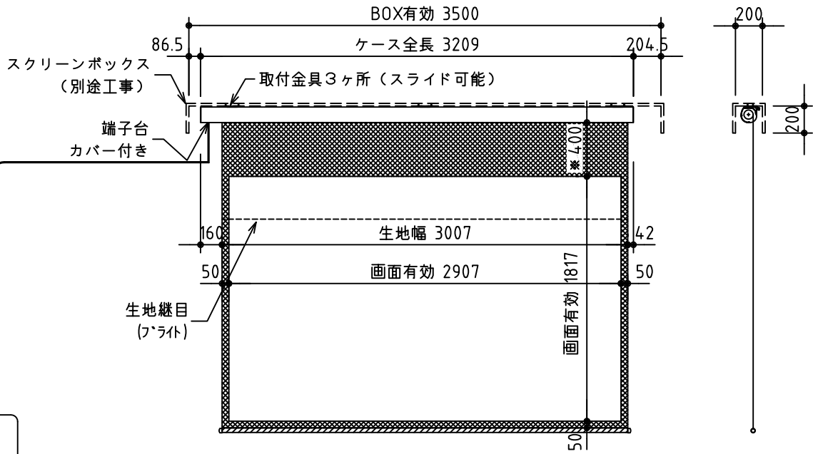
外觀図 S=1/40
