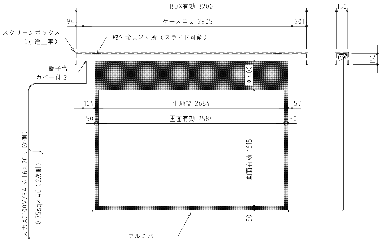
外観図 S=1/30
