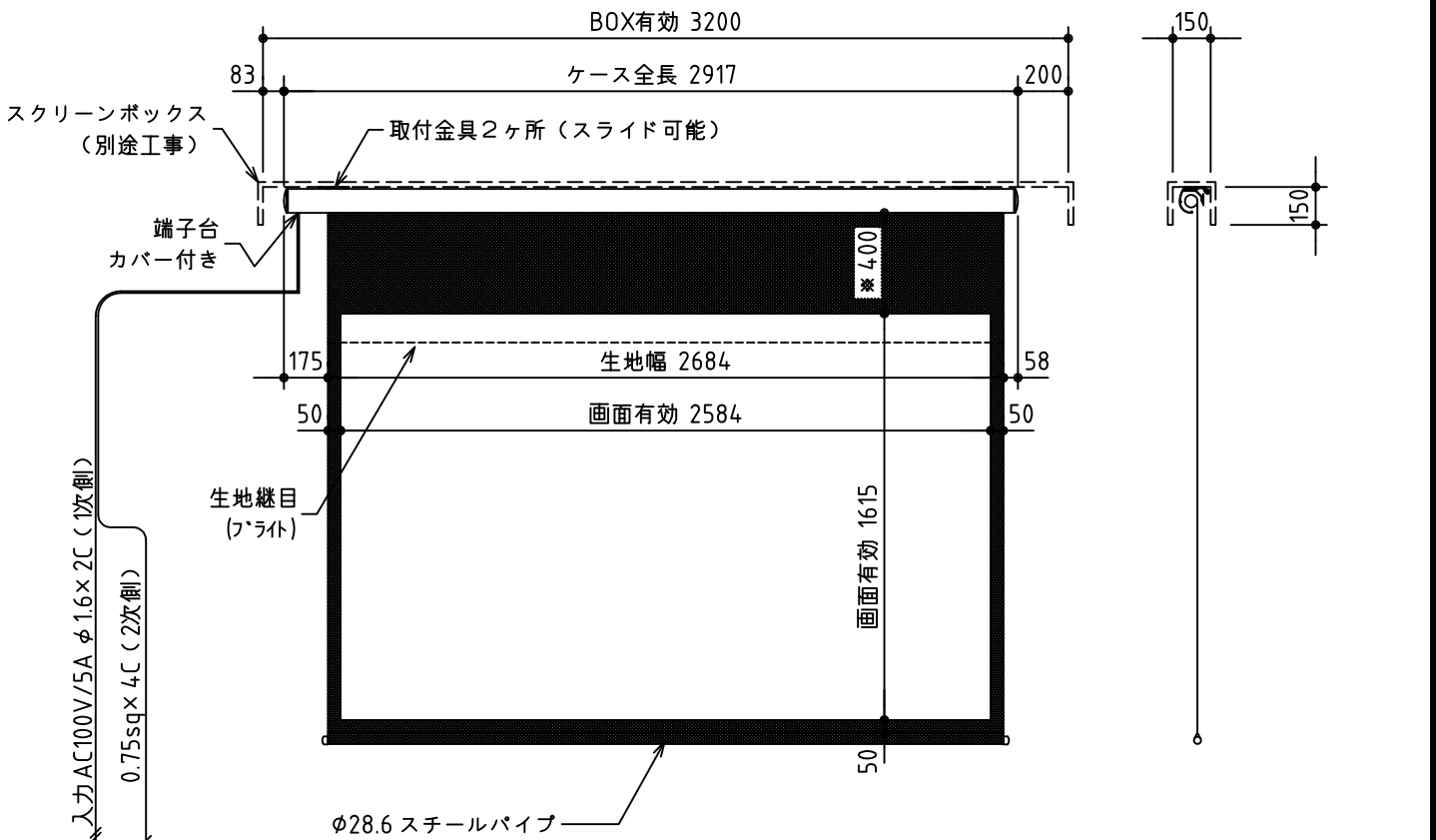
外観図 S=1/30
