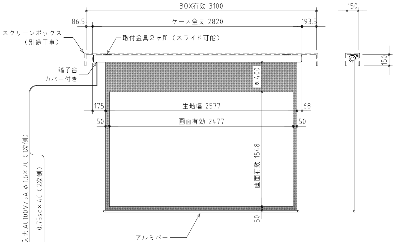
外観図 S=1/30
