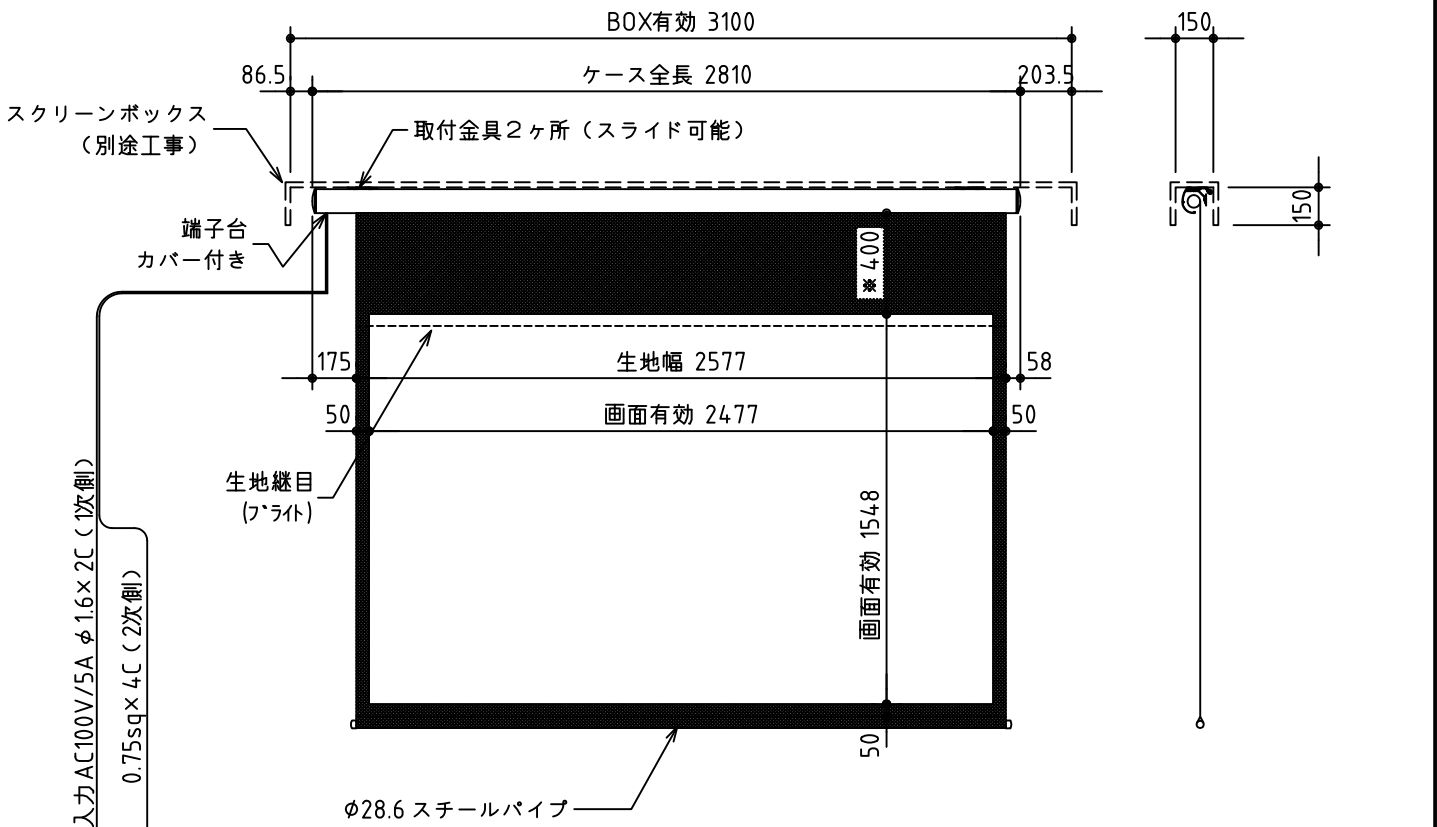
外観図 S=1/30
