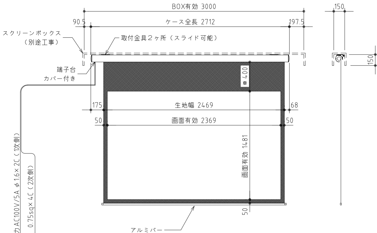
外観図 S=1/30
