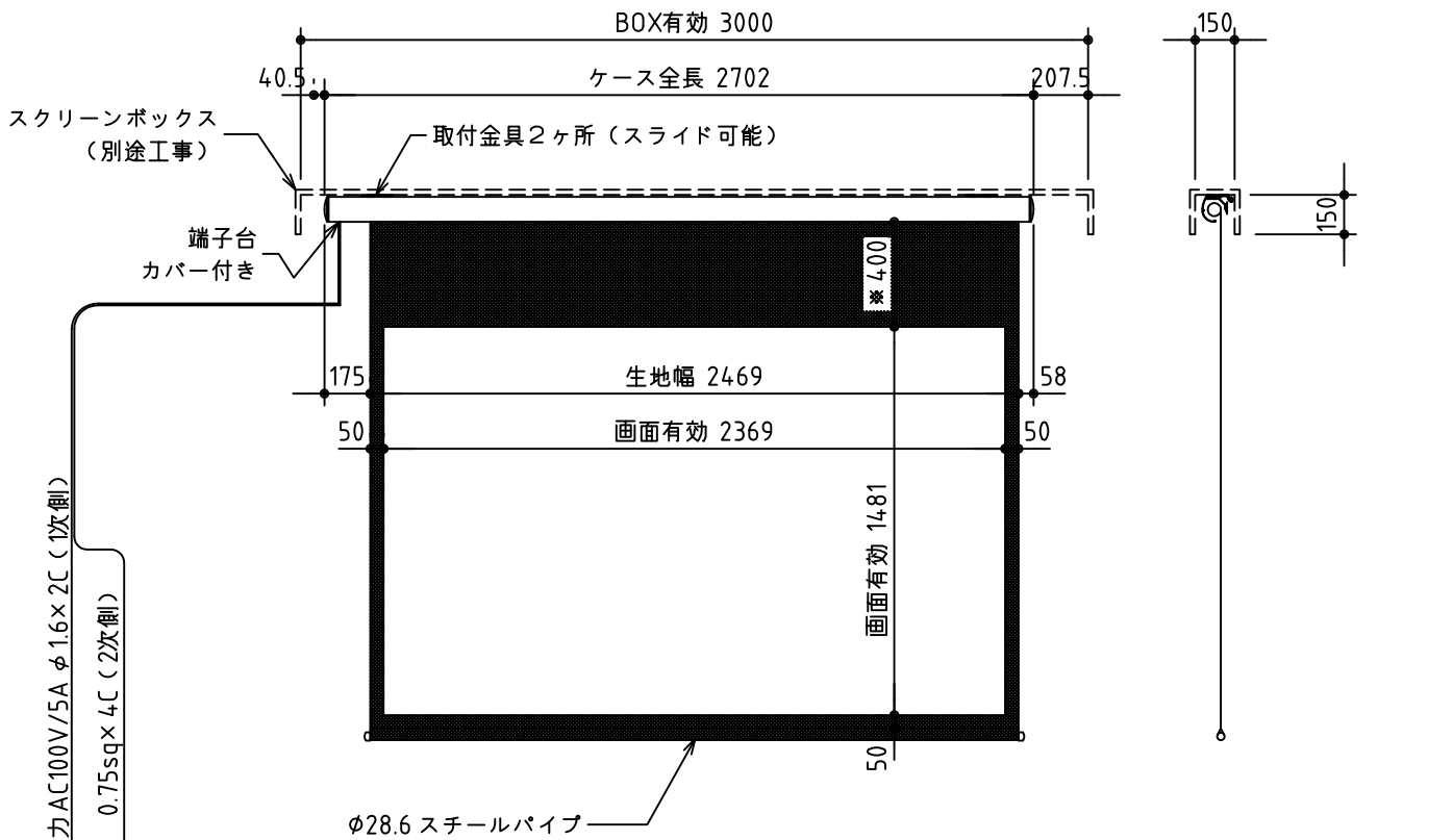
外観図 S=1/30
