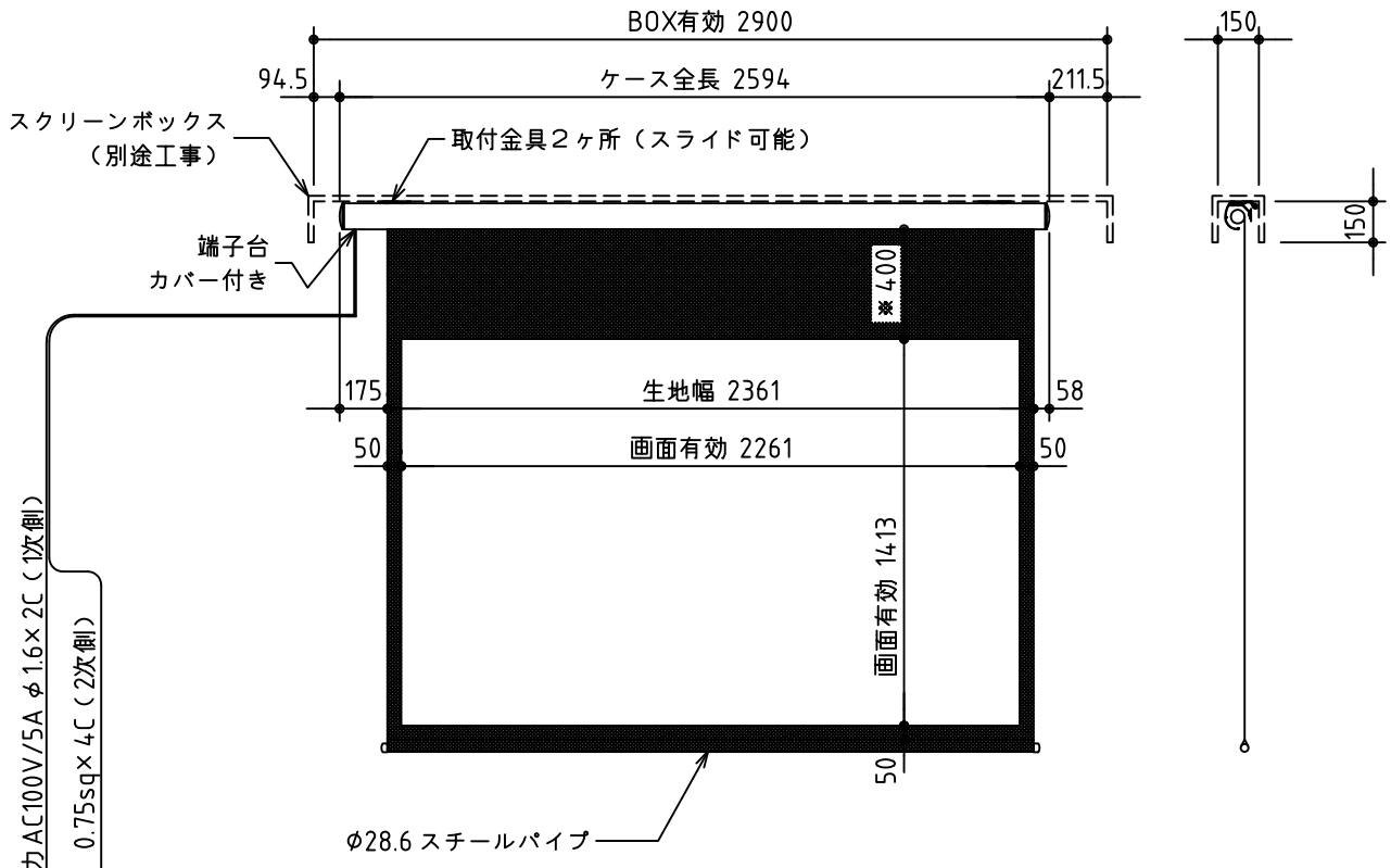
外観図 S=1/30
