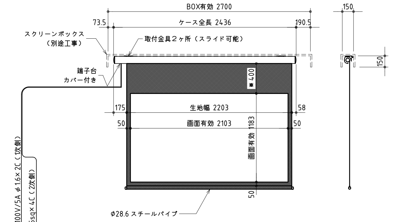
外觀図 S=1/30
