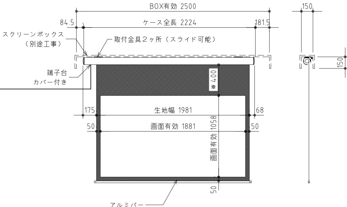
外観図 S=1/30
