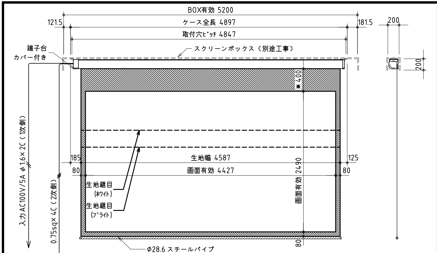
外觀図 S=1/40
