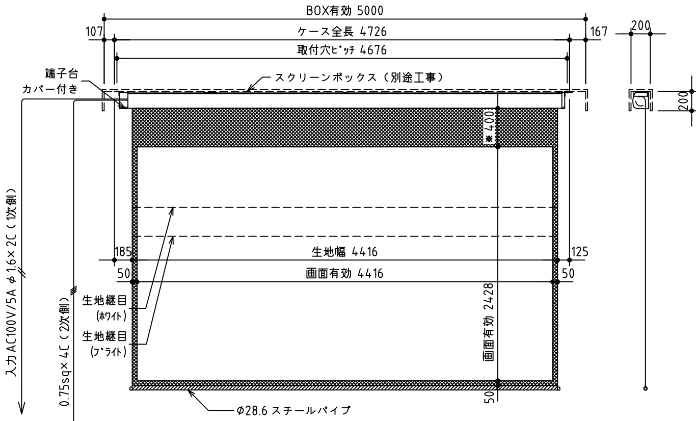
外観図 S=1/40
