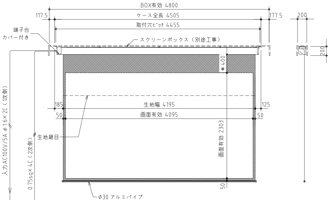
外観図 S=1/40
