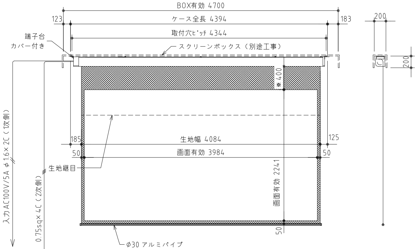
外觀図 S=1/40
