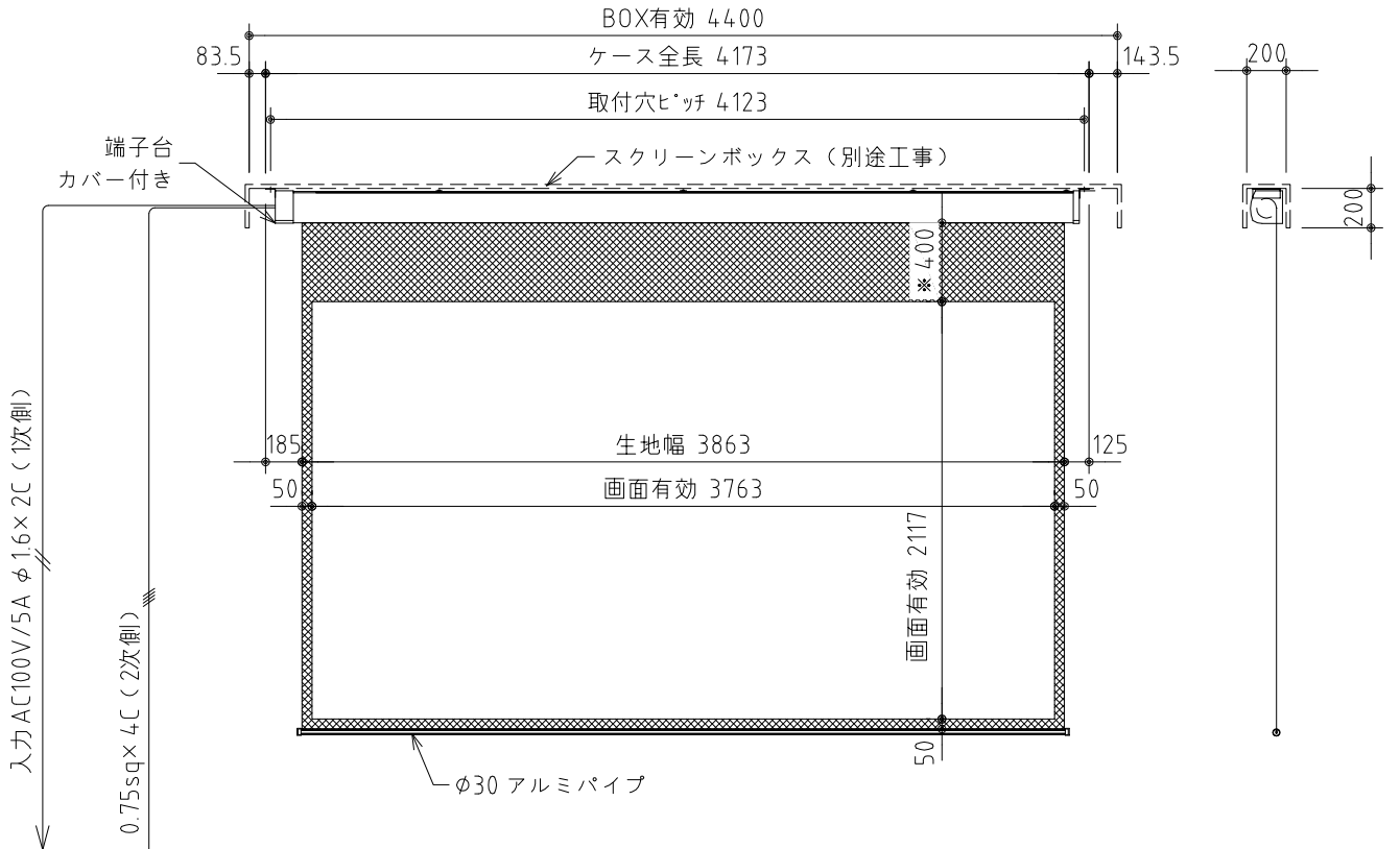
外觀図 S=1/40
