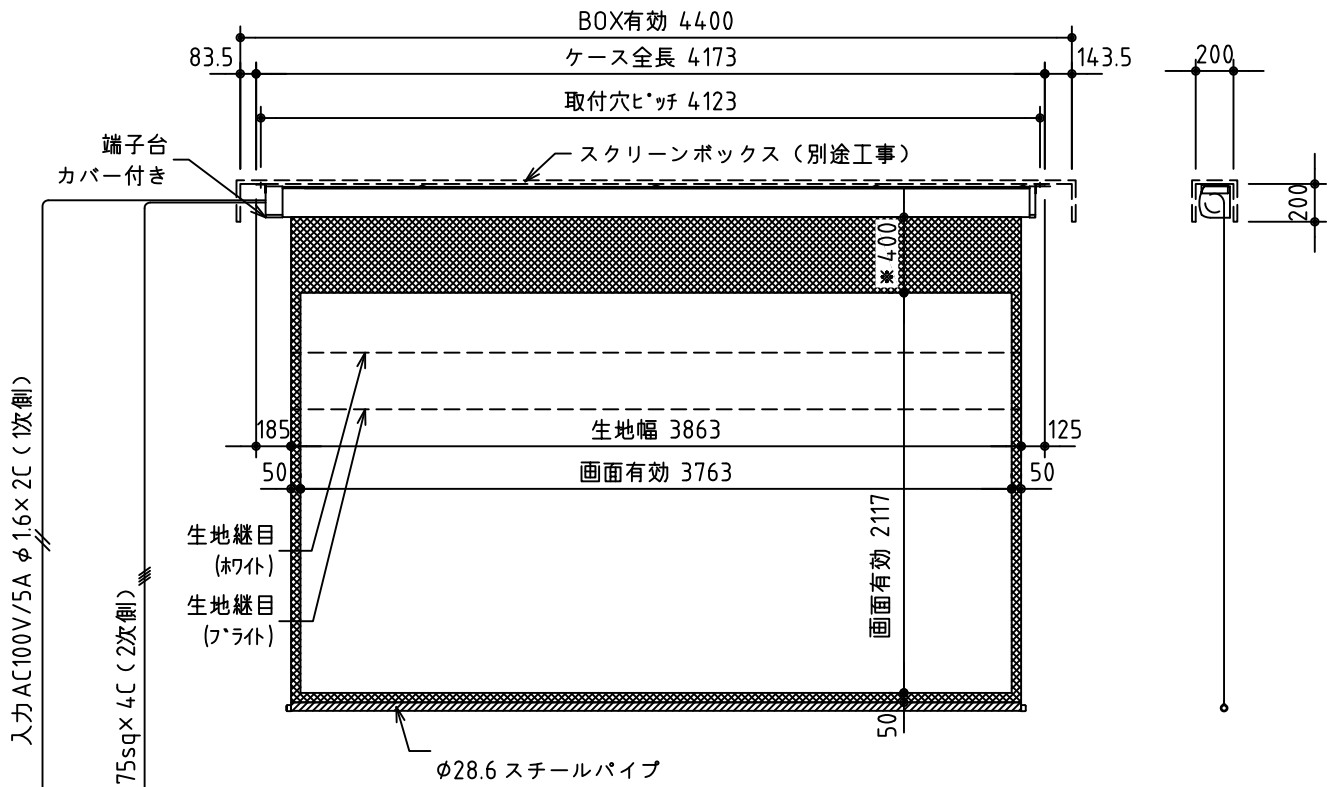
外観図 S=1/40
