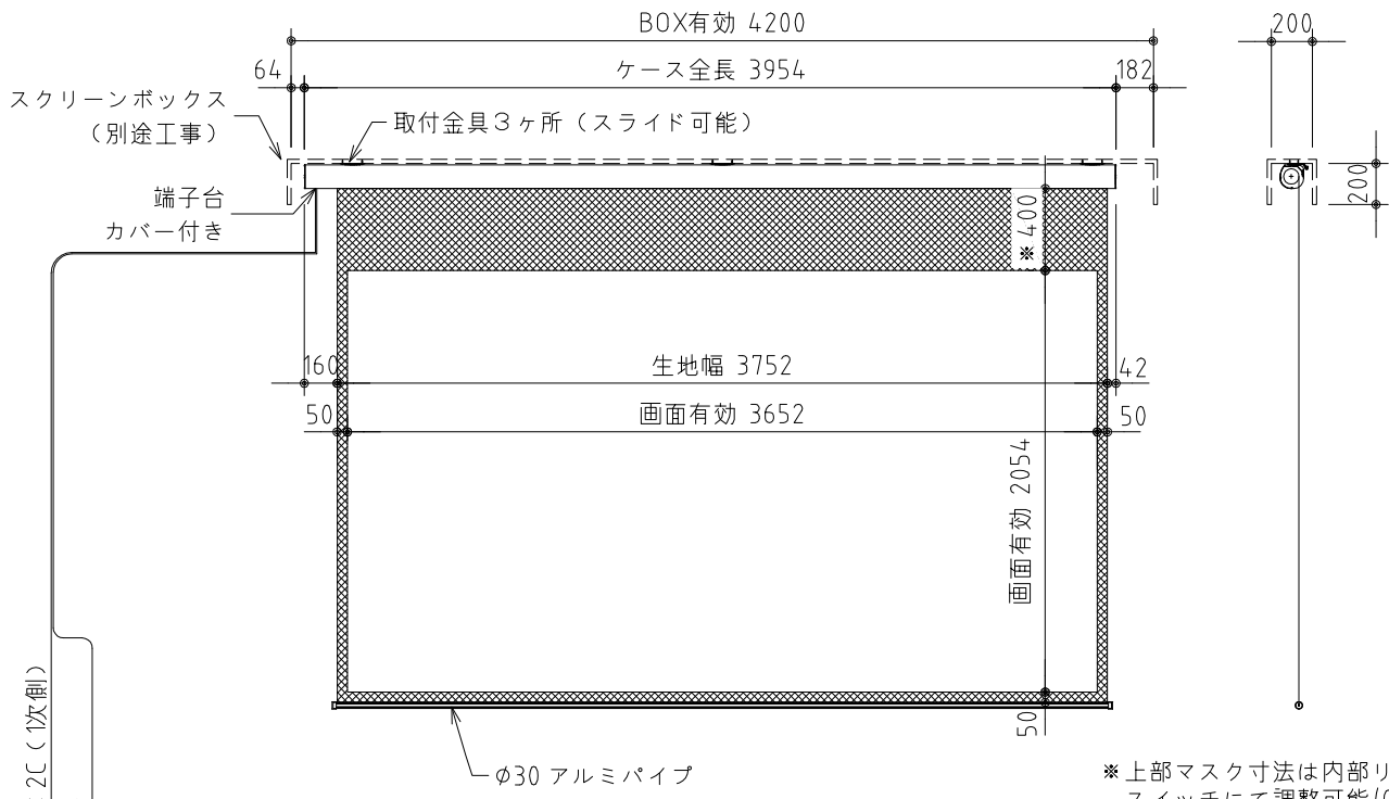
外観図 S=1/40
