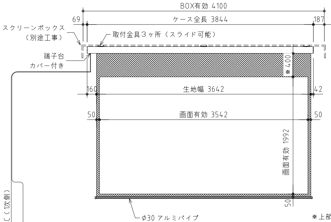
外觀図 S=1/40
