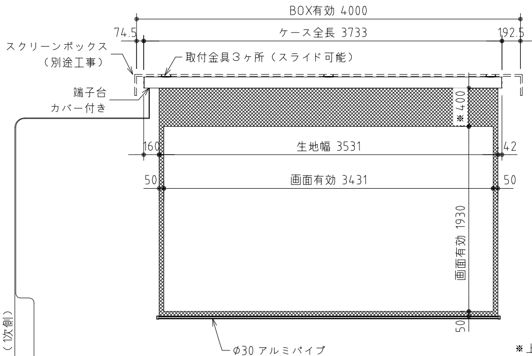
外観図 S=1/40
