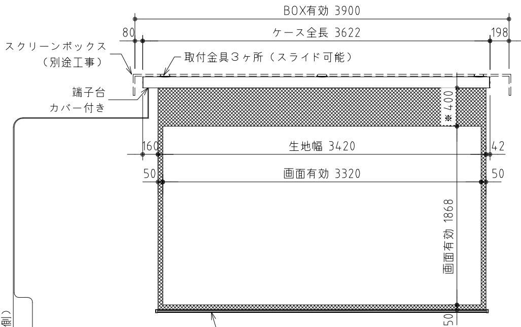
外觀図 S=1/40
