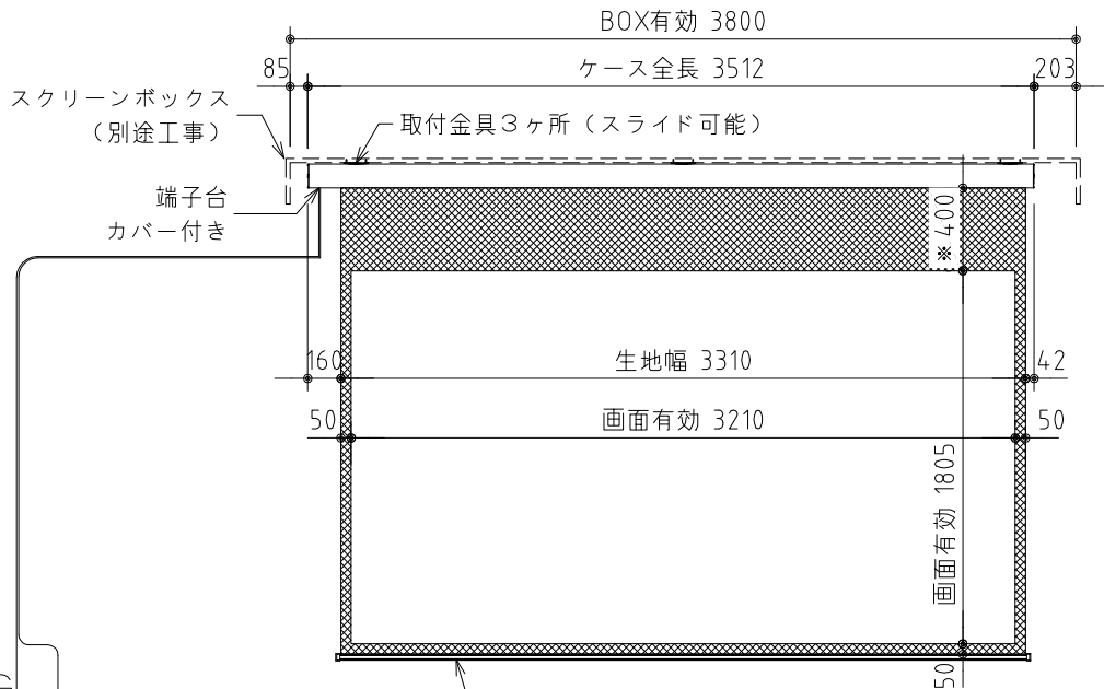
外觀図 S=1/40
