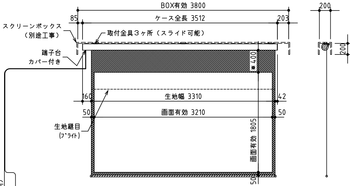
外觀図 S=1/40
