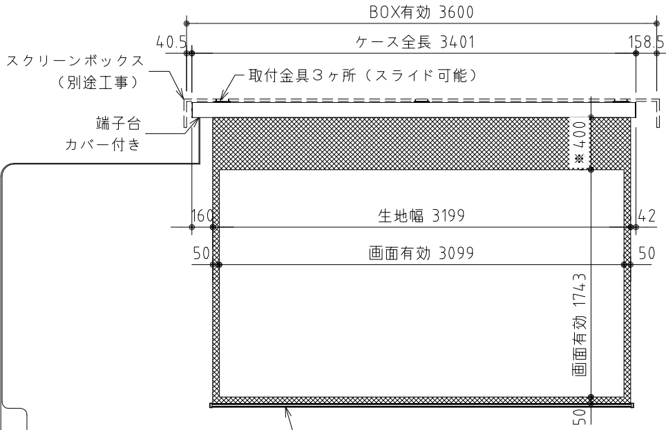
外觀図 S=1/40
