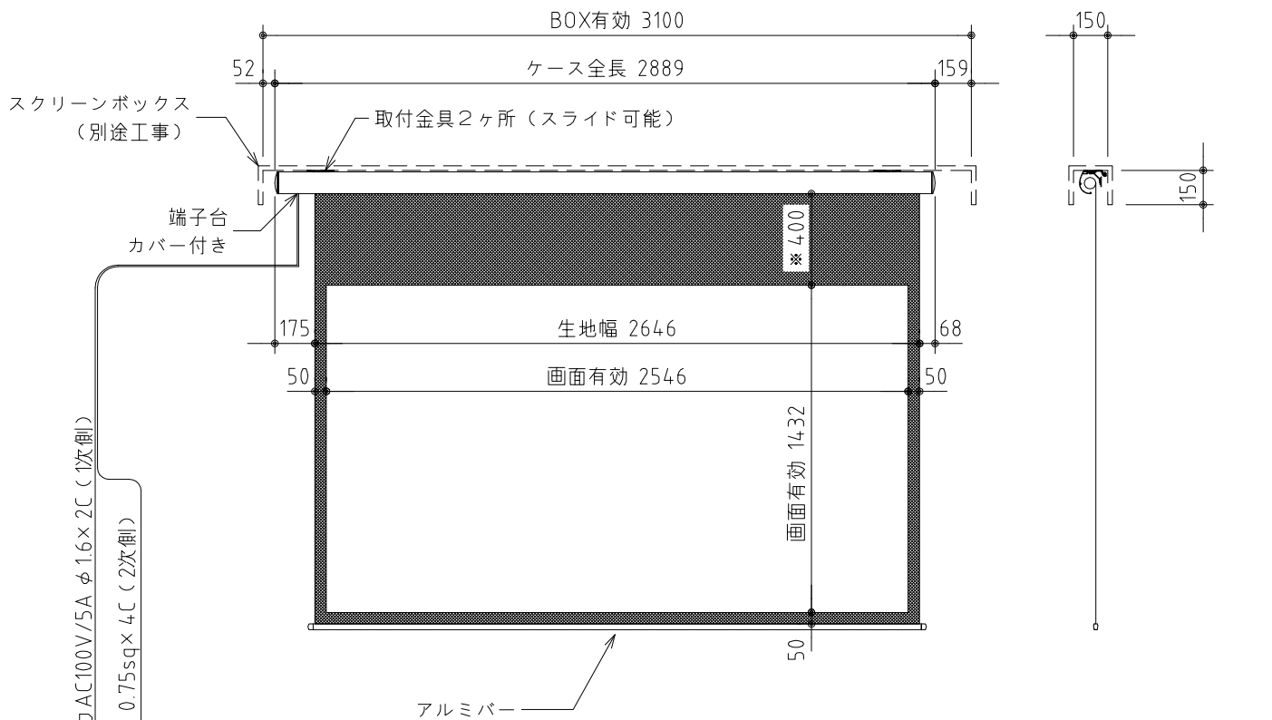
外観図 S=1/30
