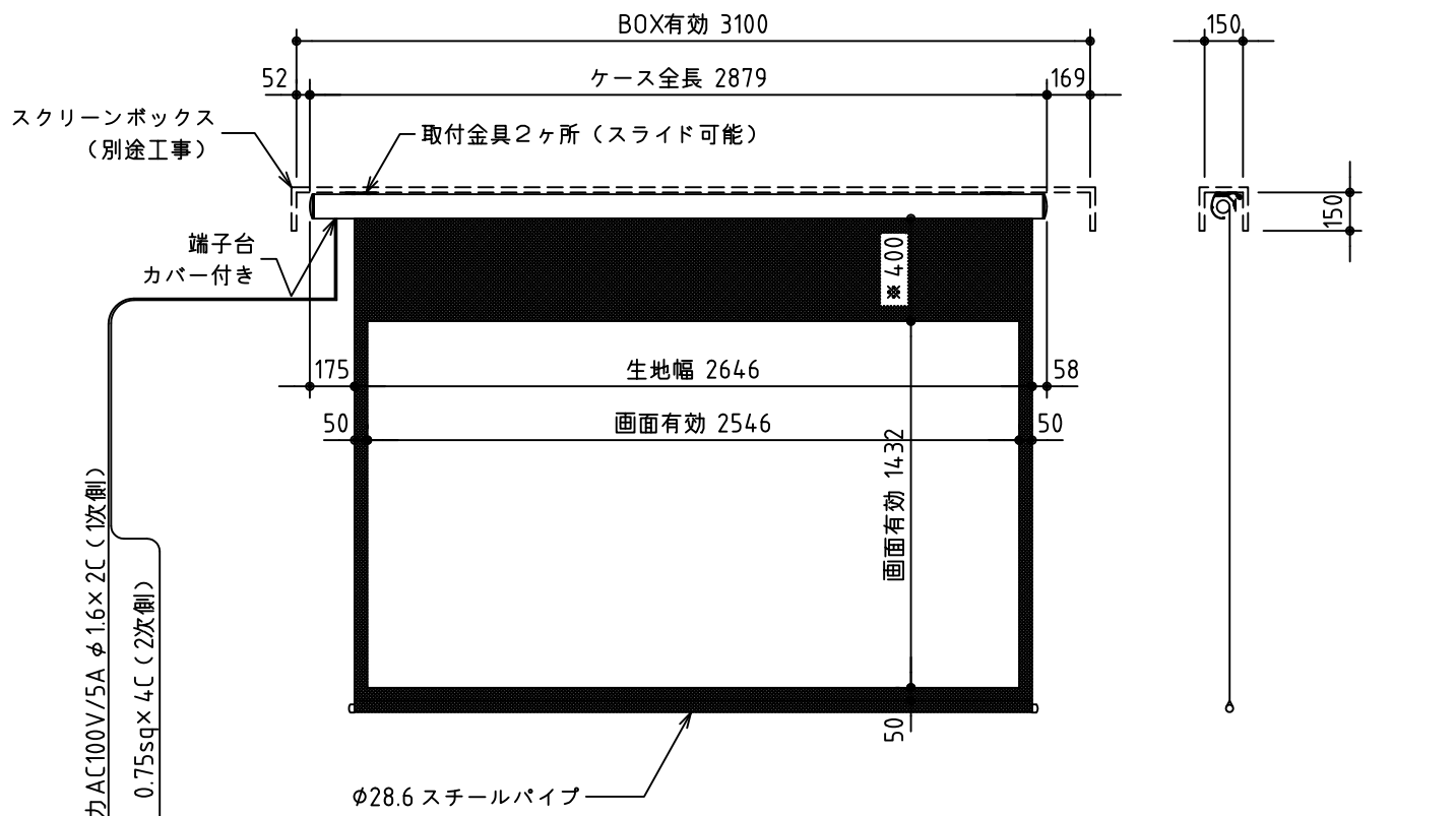
外観図 S=1/30
