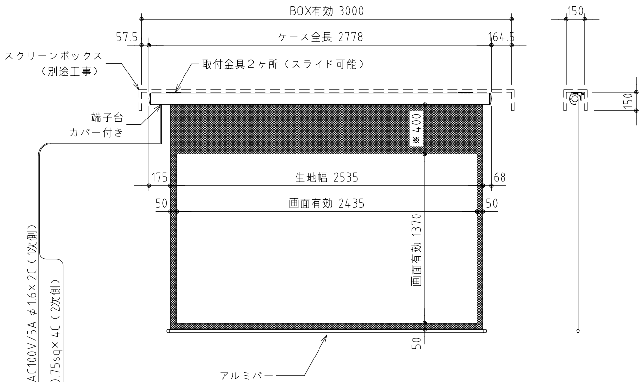
外観図 S=1/30
