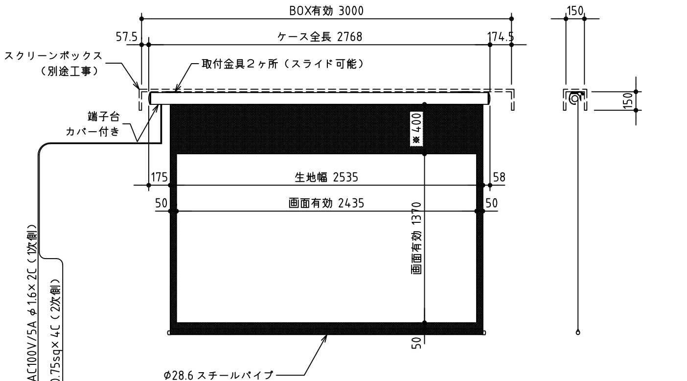
外觀図 S=1/30
