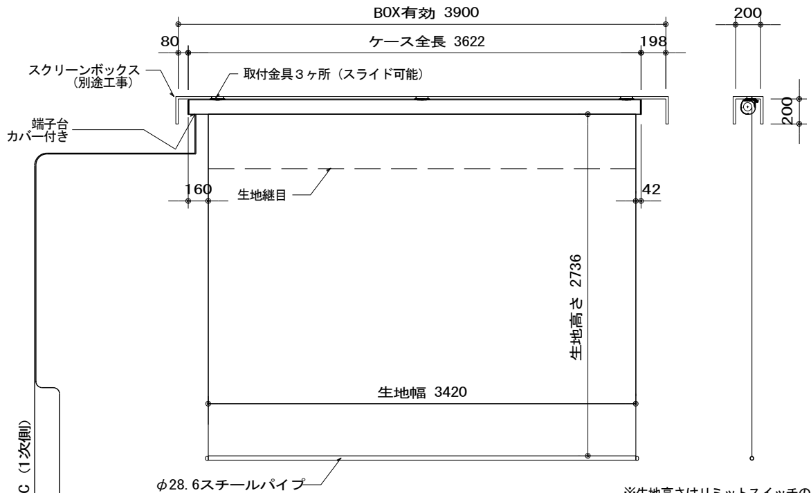
外観図 S=1/40
