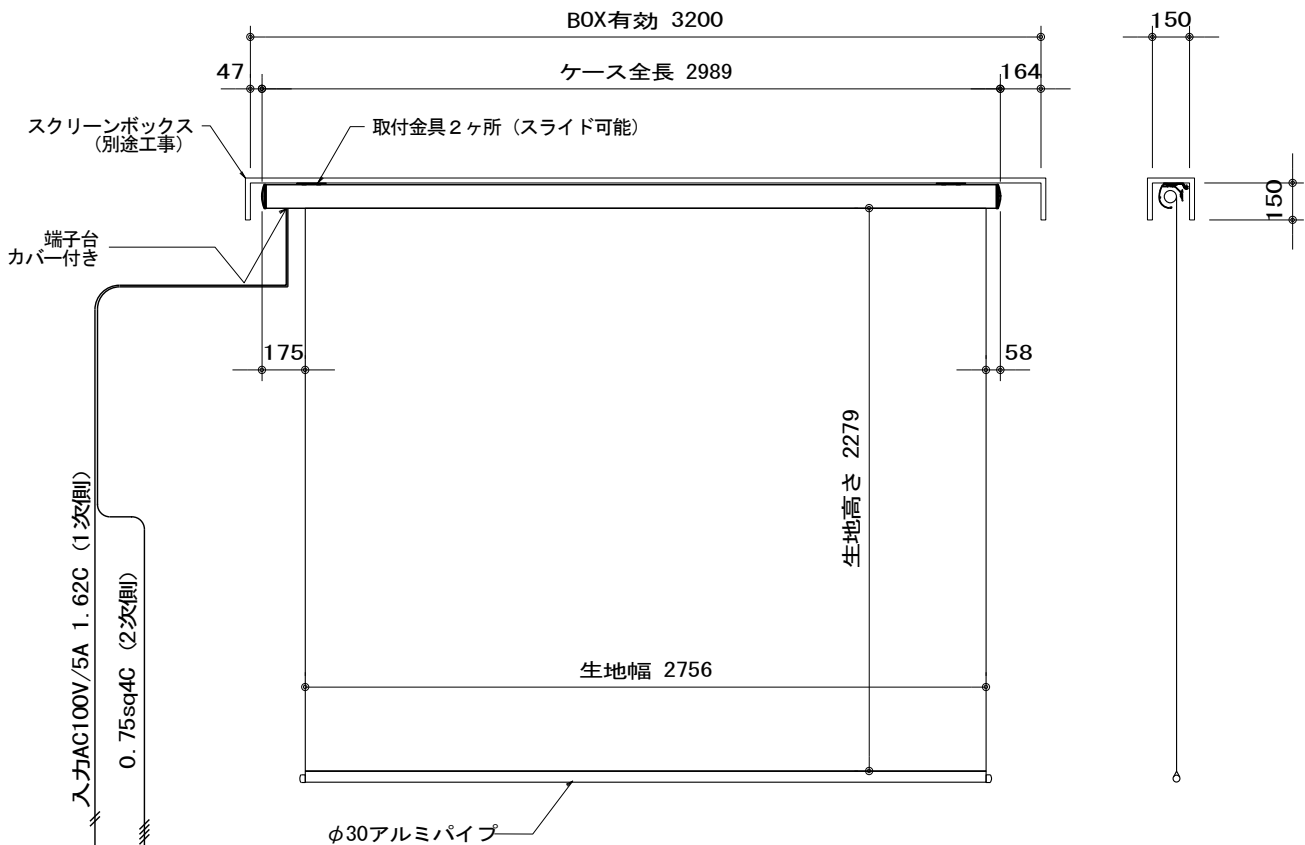
外観図 S=1/30
