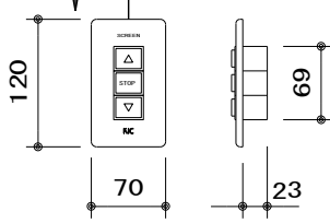
1連フルカラー埋め込みスイッチ
