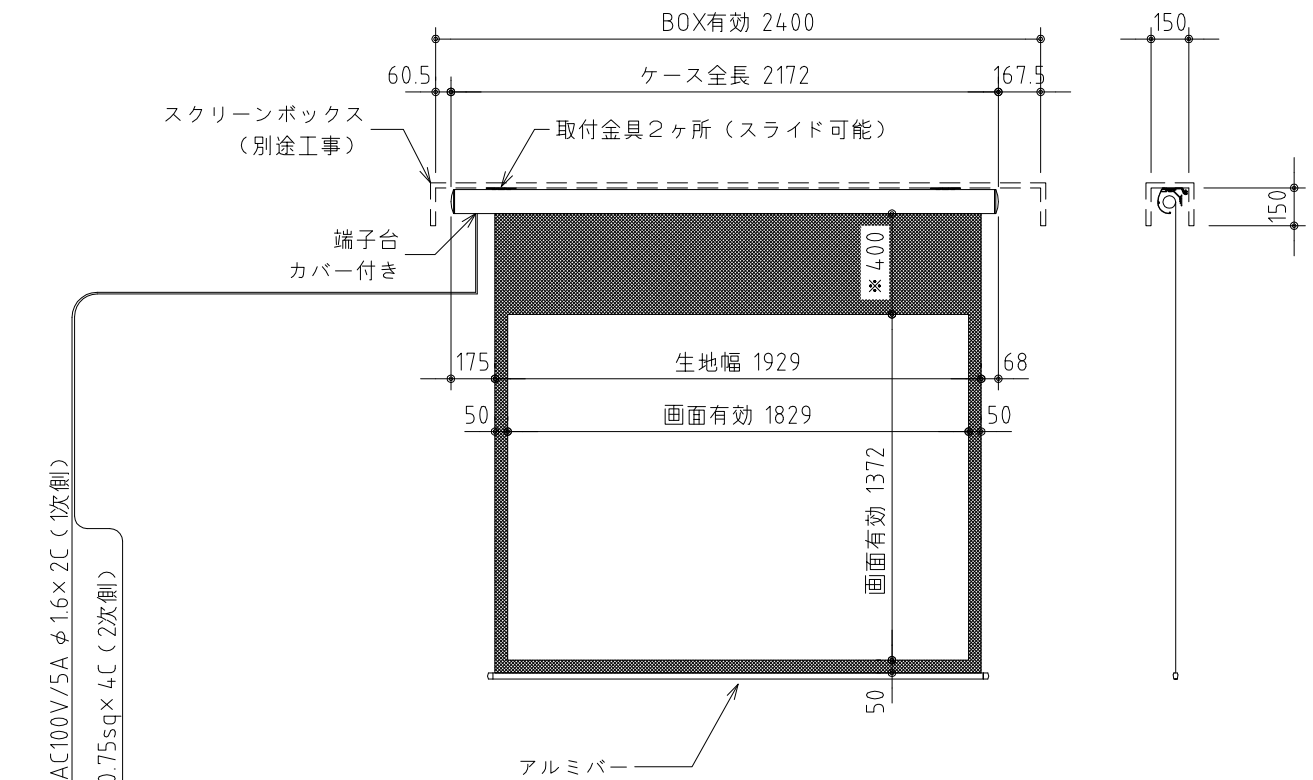
外観図 S=1/30
