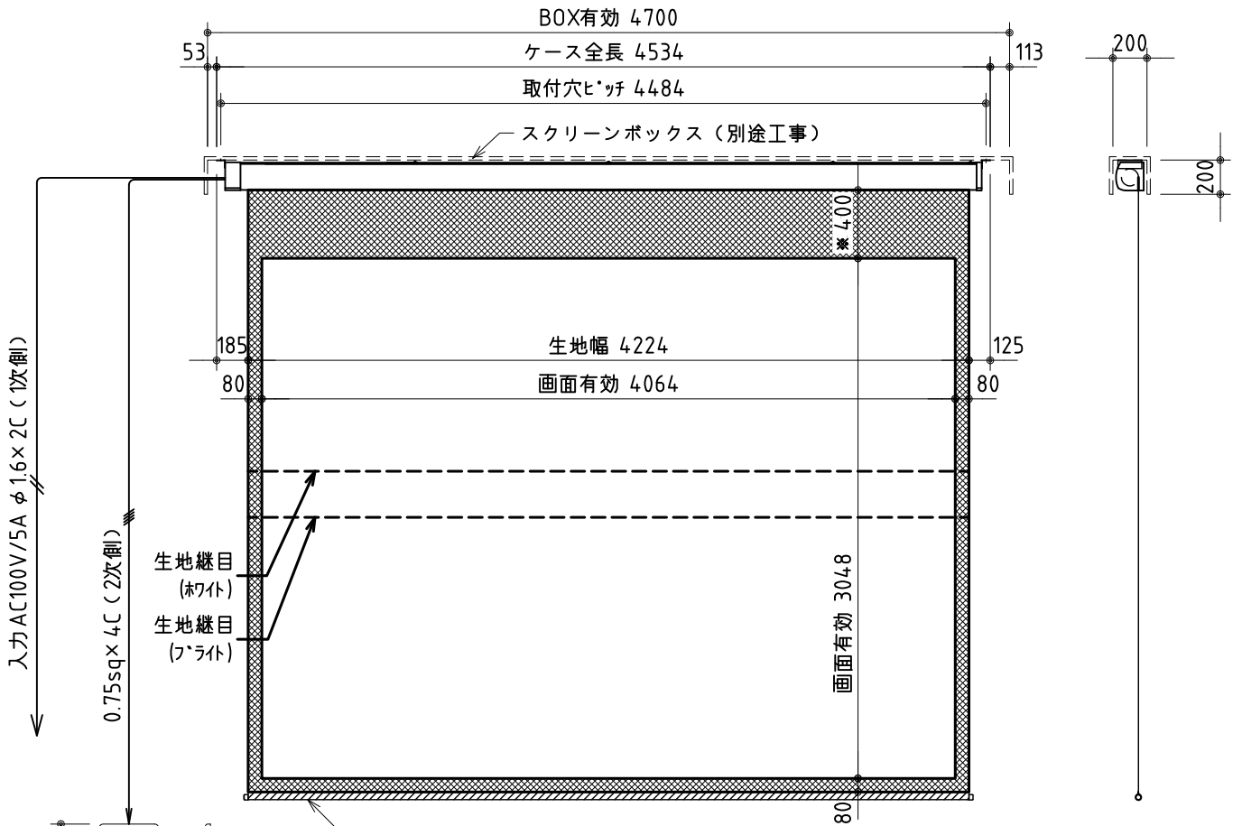
外觀図 S=1/40
