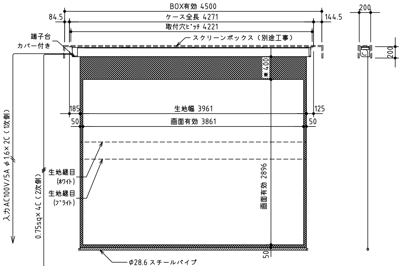
外観図 S=1/40
