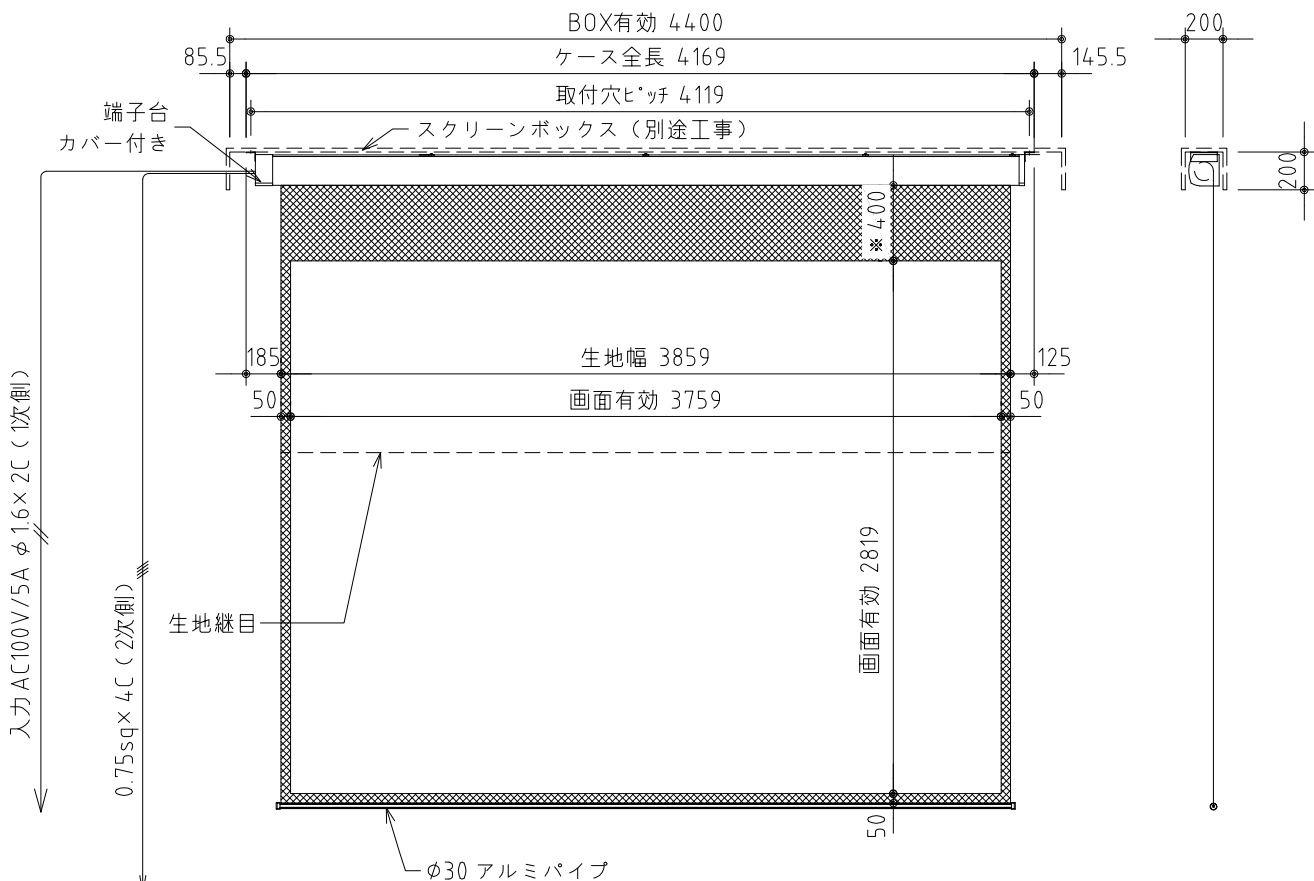
外観図 S=1/40
