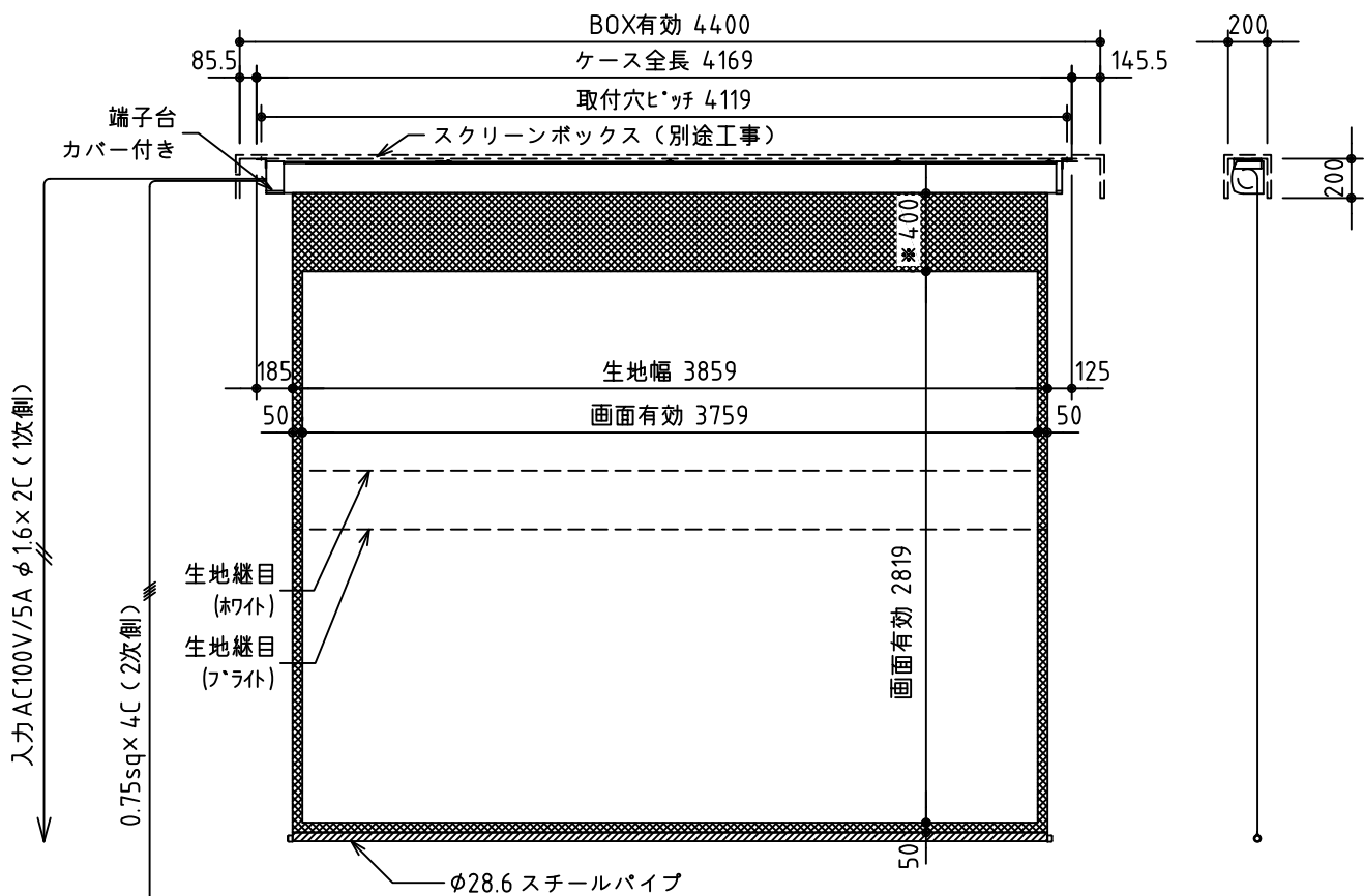
外観図 S=1/40
