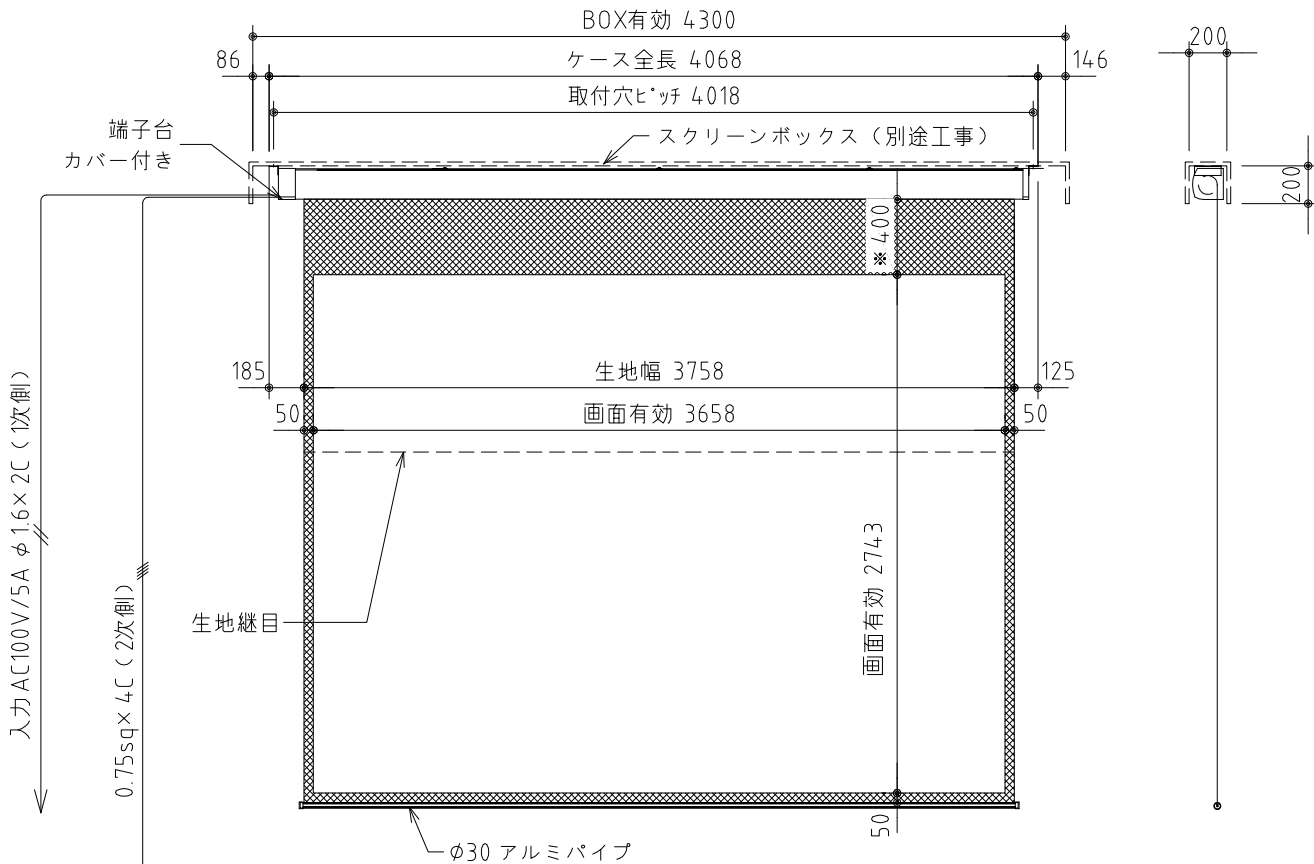
外観図 S=1/40
