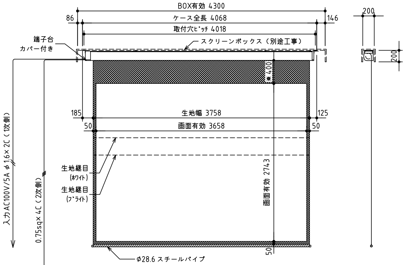
外観図 S=1/40
