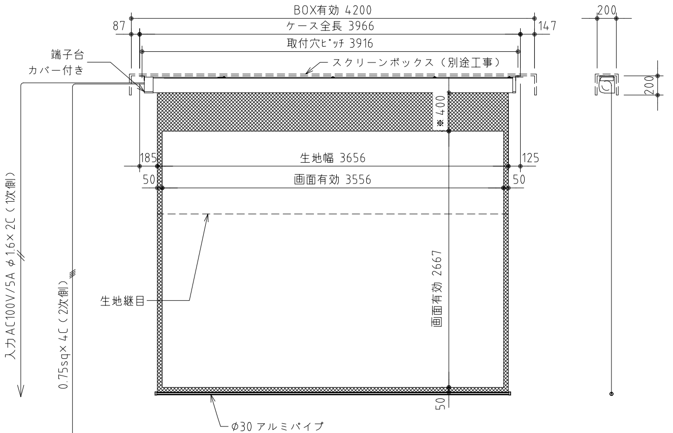
外観図 S=1/40
