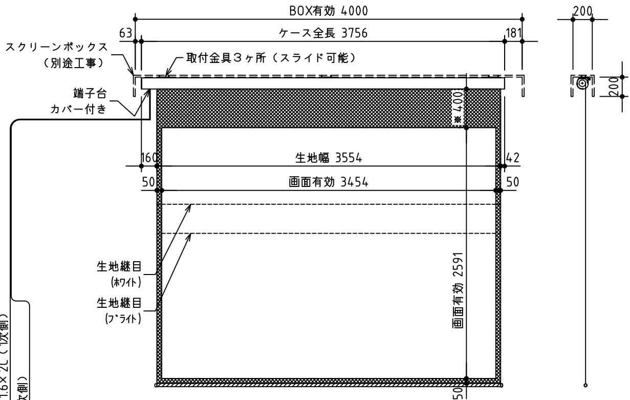
外観図 S=1/40
