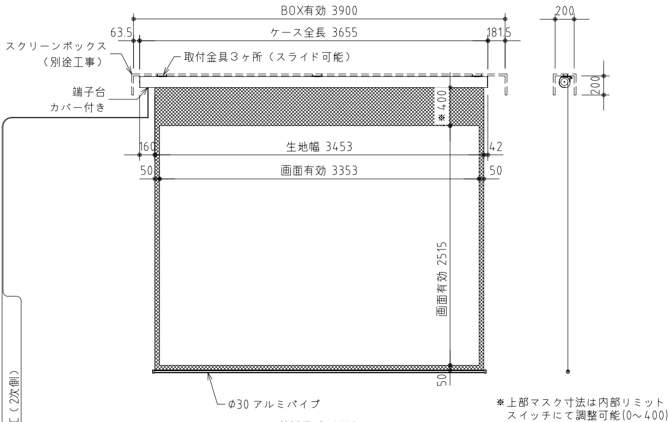
外観図 S=1/40
