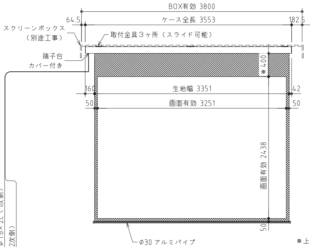
外觀図 S=1/40
