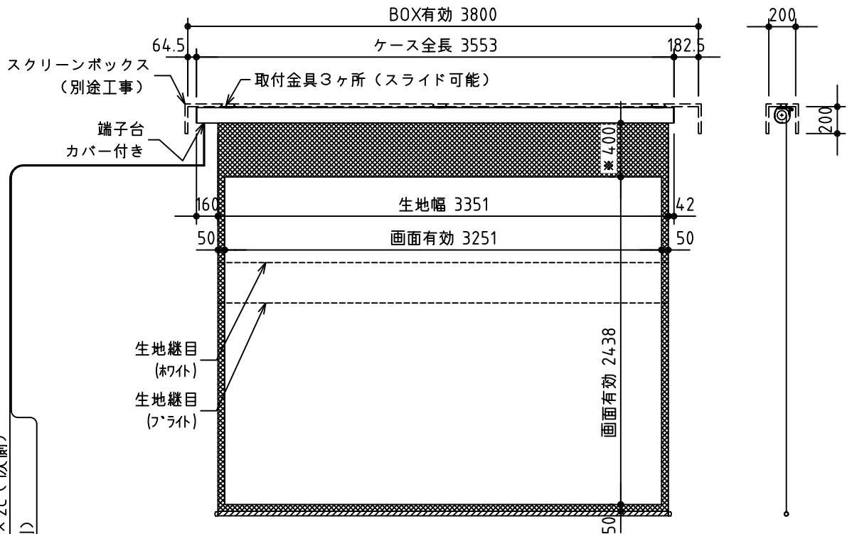
外観図 S=1/40
