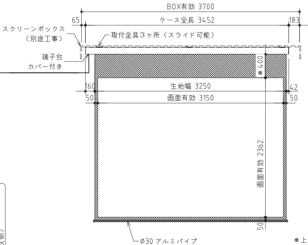
外観図 S=1/40
